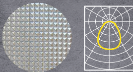
Микропризма 90^\circ
